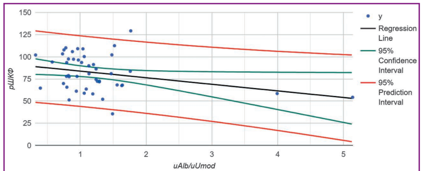
Рисунок 4. Кореляція між uAlb/uUmod і рШКФ (1-ша група)
